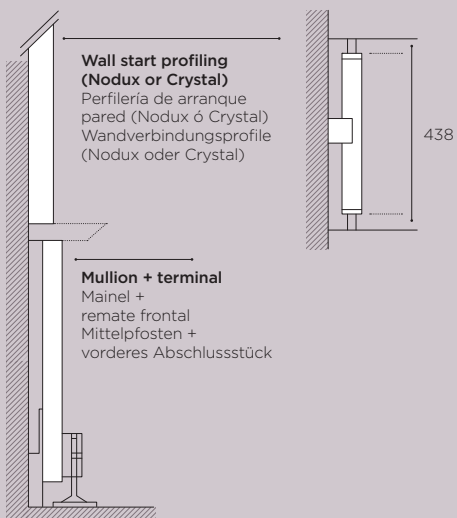
Assembly 1. Wall start. Conjunto 1. Arranque pared. Teilesatz 1: Wandverbindung.
